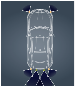
約30万画素C-MOSカメラ
