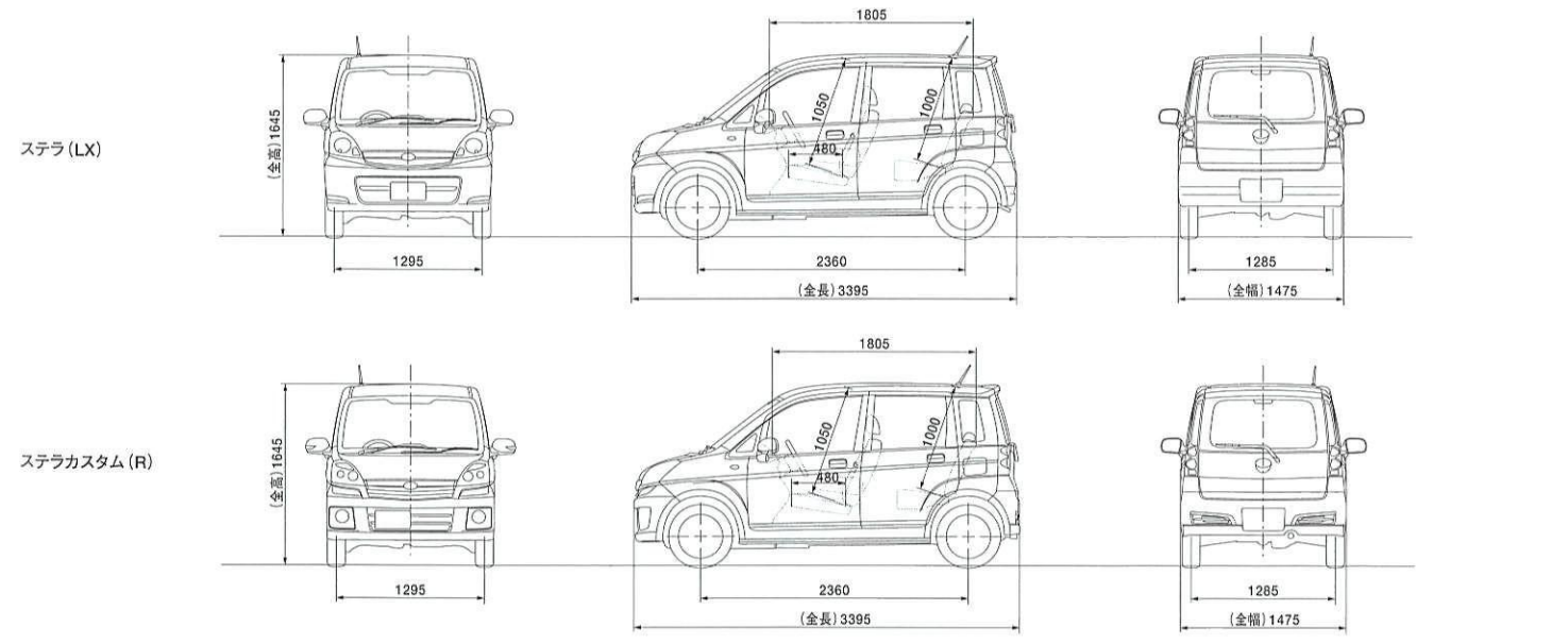
3面図 単位:mm
